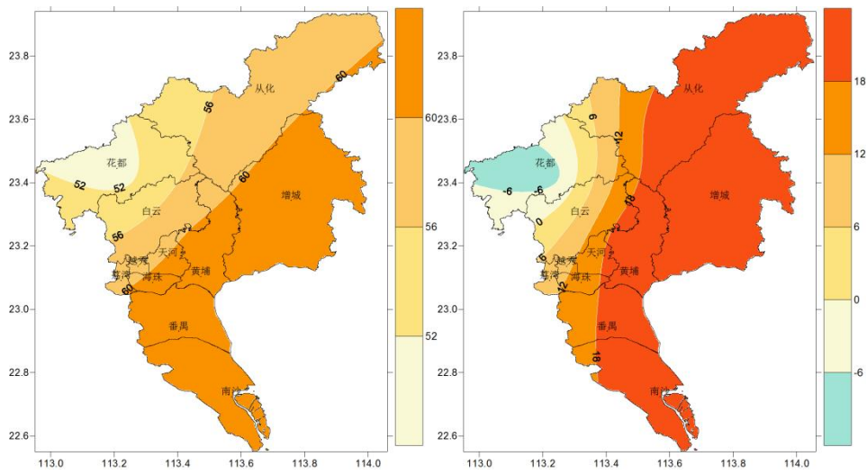
图 2 2024 年 6 月广州降水量（毫米）、降水距平百分率（%）
