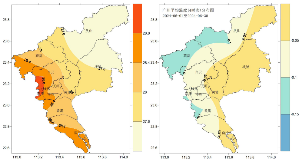
图 1 2024 年 6 月广州平均气温 (°C)、气温距平 (°C)
