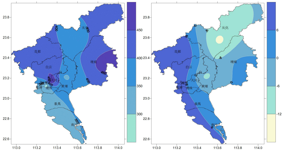
图 2 2024 年 6 月广州降水量（毫米）、降水距平百分率（%）
