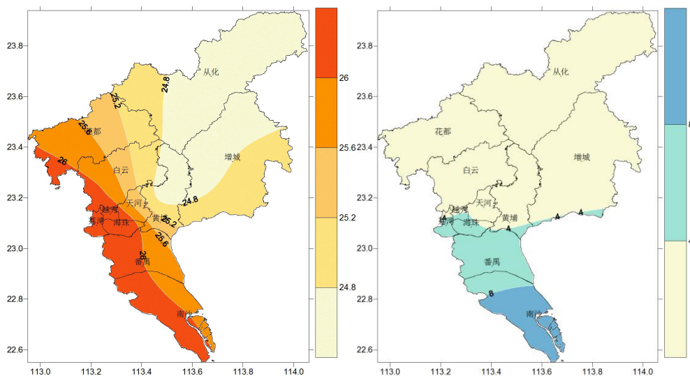
图 1 2023 年 10 月 23 日~10 月 30 日广州市日平均气温（左图，单位： ^{\circ}\text{C} ） 和累计降雨量（右图，单位：毫米）分布图
