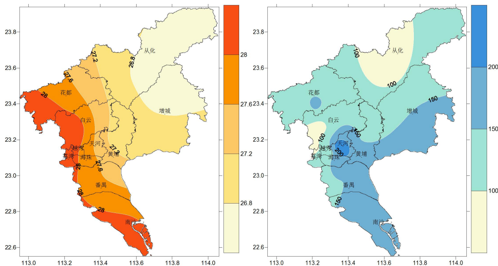
图 1 2023 年 6 月 13 日~6 月 19 日广州市平均气温（左图，单位：℃）和 累计降雨量（右图，单位：毫米）分布图
