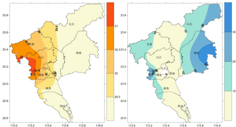
图 1 2022 年 6 月 23 日~6 月 29 日广州市日平均气温（左图，单位： ^{\circ}\text{C} ） 和累计降水量（右图，单位：毫米）分布图
