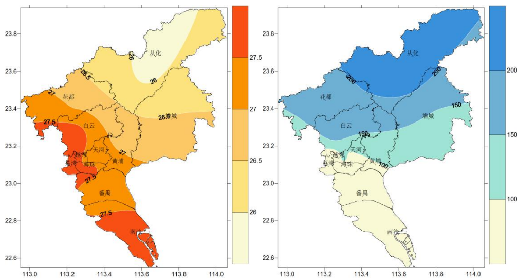
图 1 2022 年 6 月 13 日~6 月 19 日广州市日平均气温（左图，单位：℃） 和累积降水量（右图，单位：毫米）分布图
