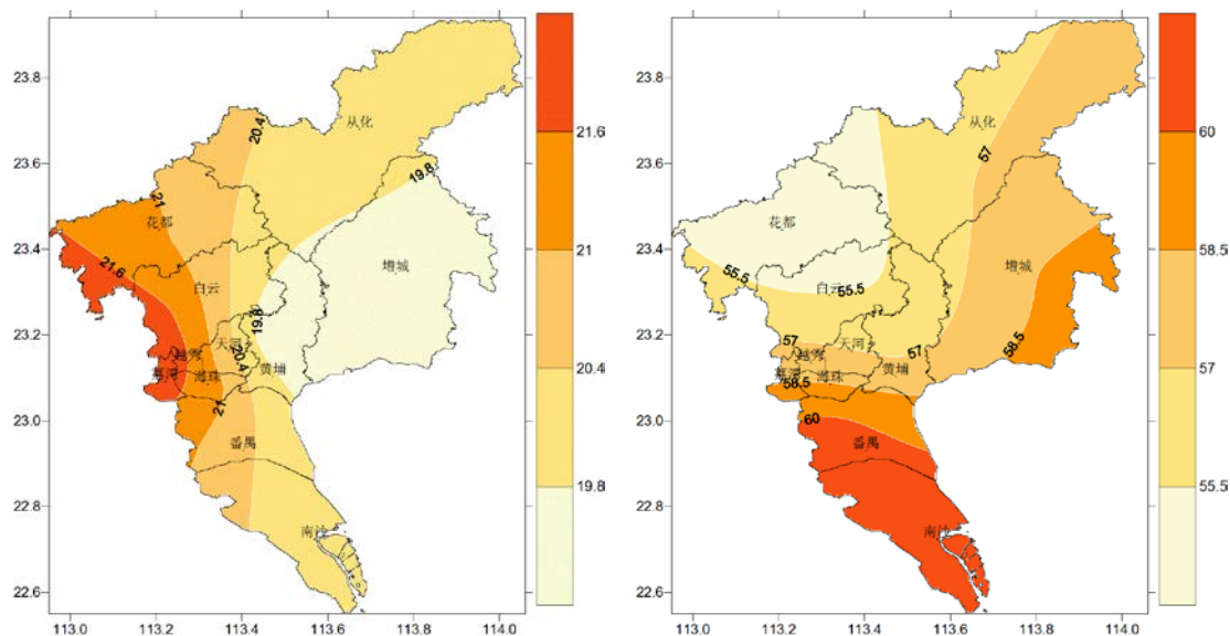
图1 2022年3月4日~3月10日气温（左图，单位： ^{\circ}\text{C} ）和累计日照时数（右图，单位：小时）分布图
