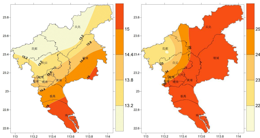
图1 2022年2月9日~2月15日广州市日平均气温（左图，单位： ^{\circ}\text{C} ）和累积日照时数（右图，单位：小时）分布图
