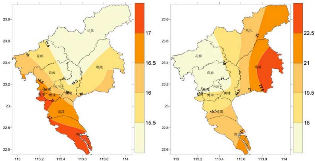
图1 2022年1月17日~1月23日广州市日平均气温（左图，单位：℃）
