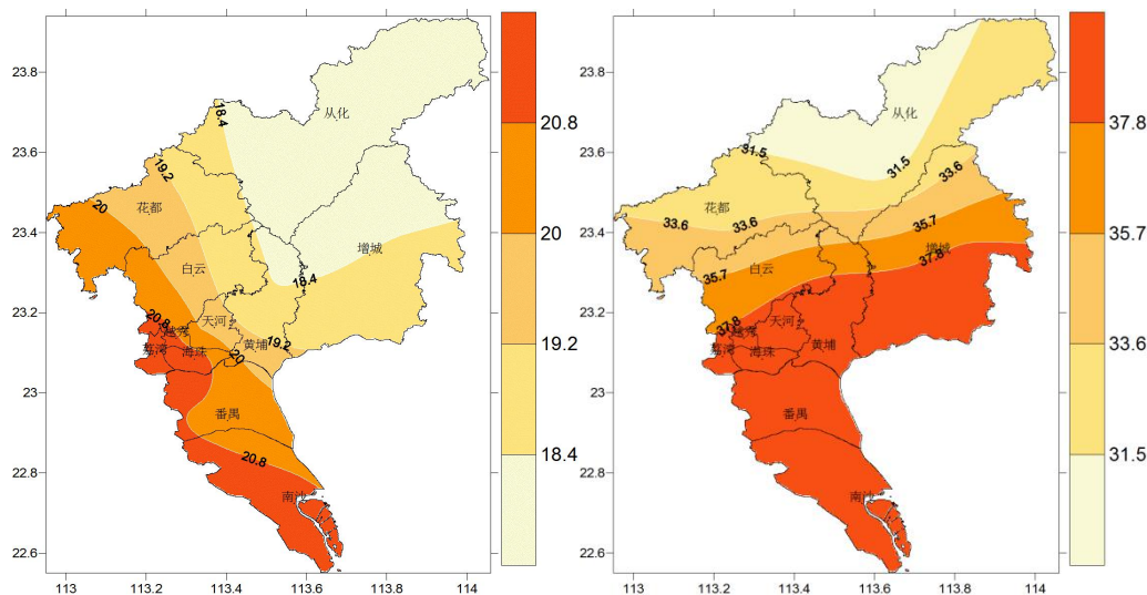
图 1 2021 年 11 月 12 日~11 月 18 日平均气温（左图，单位： ^{\circ}\text{C} ）和累积日照时数（右图，单位：小时）分布图
