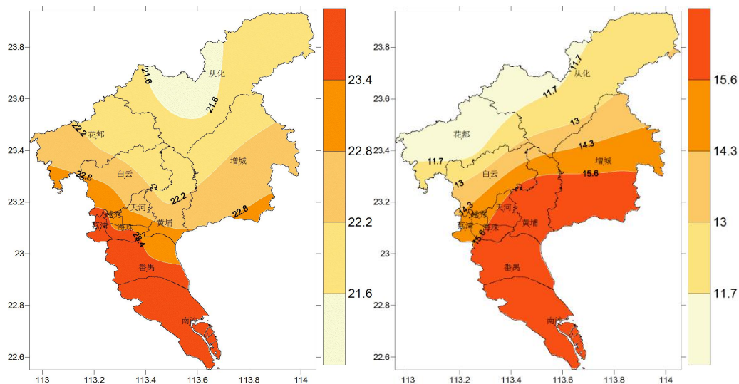
图1 2021年10月29日~11月4日气温（左图，单位：℃）和累计日照时数（右图，单位：小时）分布图
