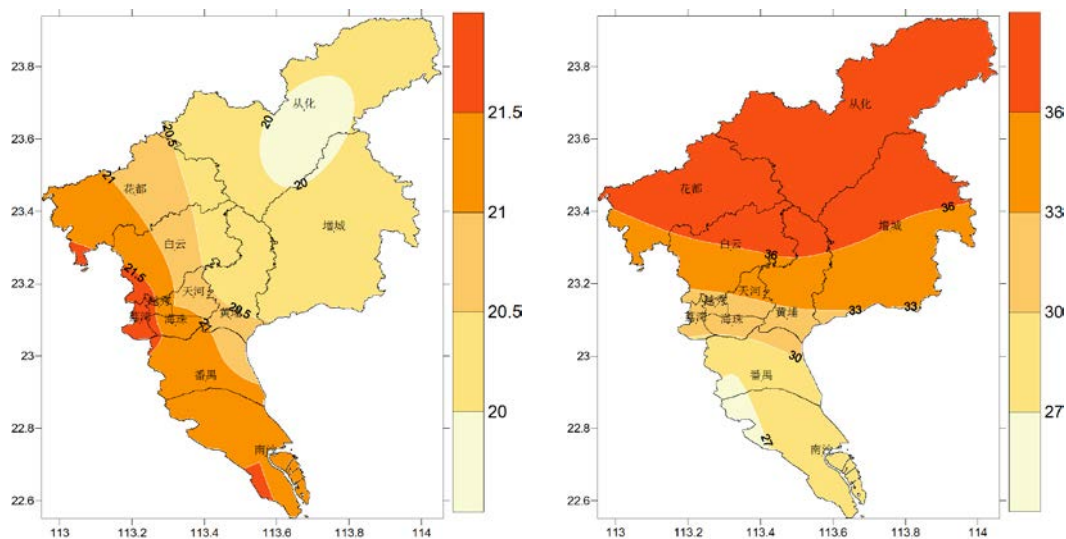
图1 2021年10月22日~10月28日气温（左图，单位： ^{\circ}\text{C} ）和累计日照时数（右图，单位：小时）分布图
