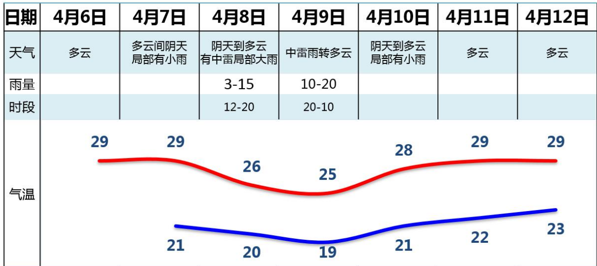
图2 广州市未来一周天气预报
