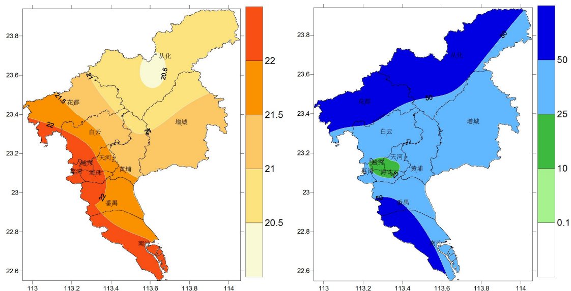
图1 2021年2月21日~4月5日气温（左图，单位： ^{\circ}\text{C} ）和累积降雨量（右图，单位： \text{mm} ）分布图
