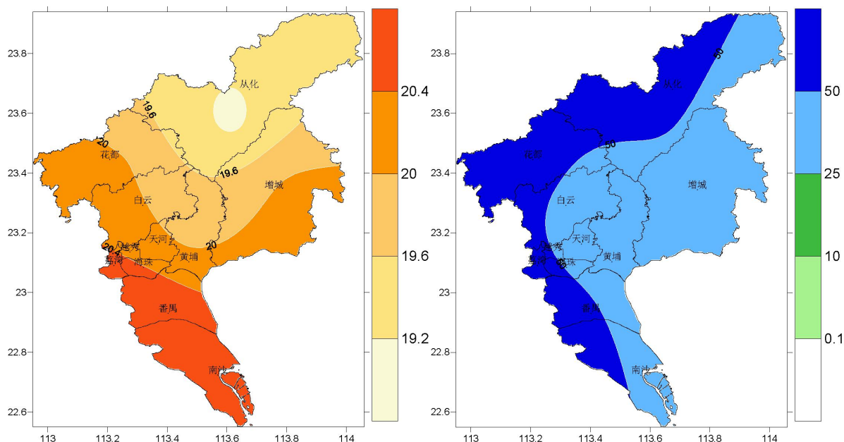
图1 2021年2月21日~3月24日气温（左图，单位： ^{\circ}\text{C} ）和累积降雨量（右图，单位： \text{mm} ）分布图
