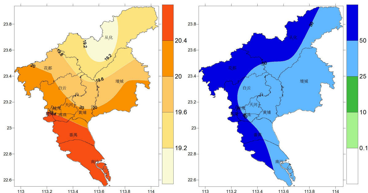
图1 2021年2月21日~3月17日气温（左图，单位： ^{\circ}\text{C} ）和累积降雨量（右图，单位： \text{mm} ）分布图
